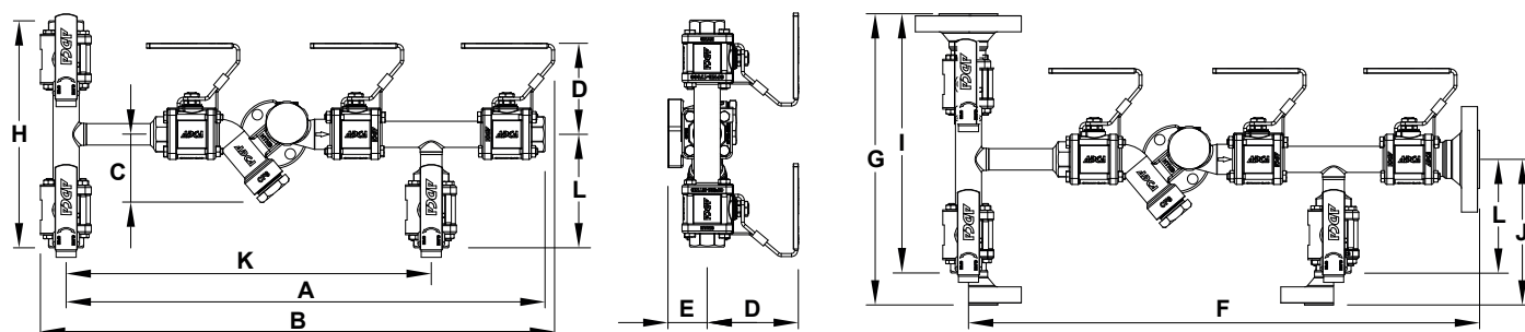
DIMENSIONS – CTS4UDB2-VH (mm)
