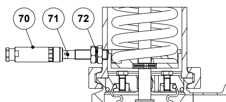
Indicador de elevación opcional
