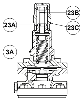
Optional top cap
