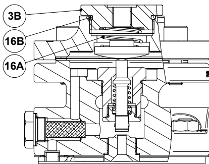
Optional dome-loading
