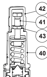
Optional top cap
