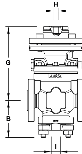
Optional dome-loading
