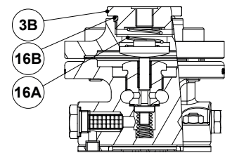
Optional dome-loading
